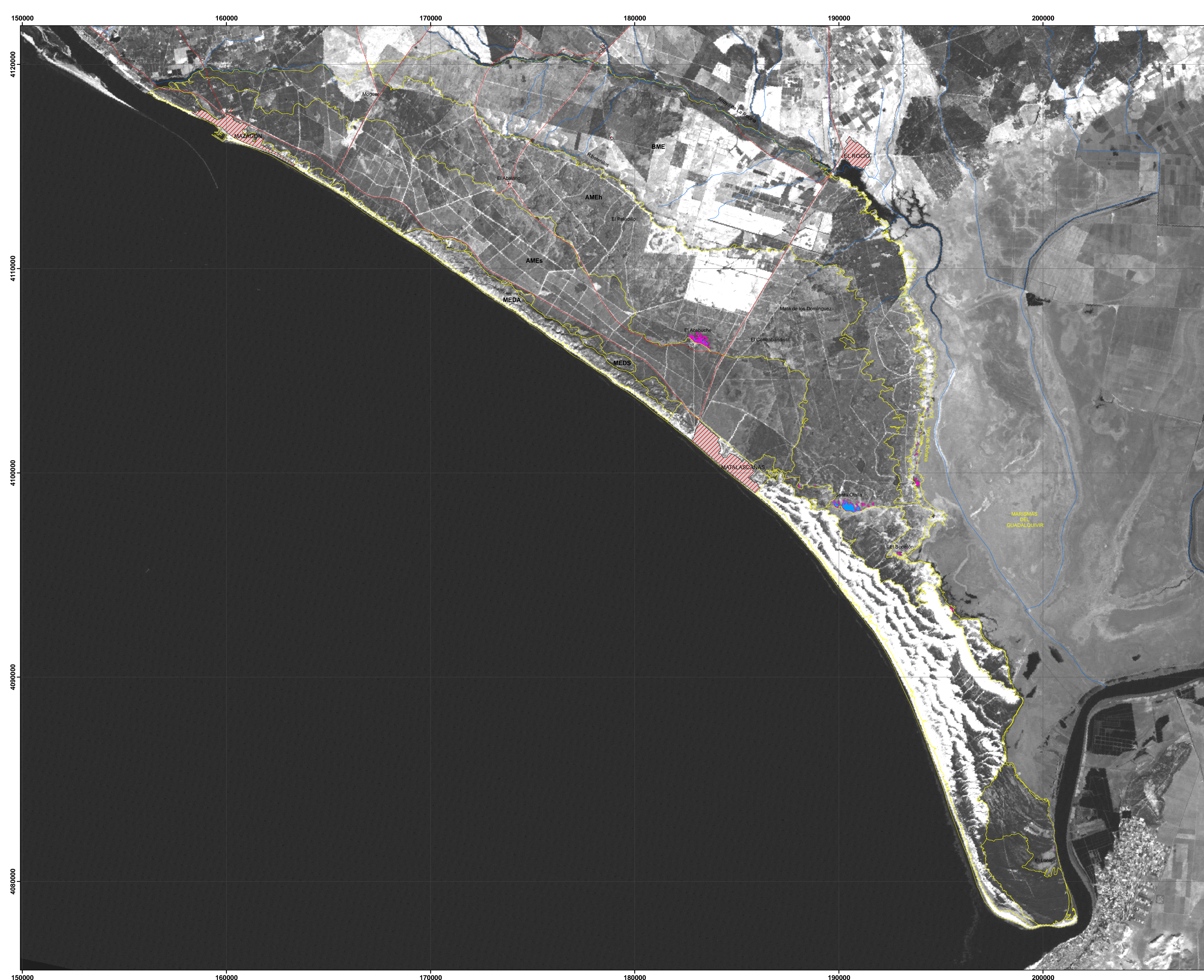
Cartografía de lámina de agua y superficies encharcadas. Enero 1999. Landsat TM
